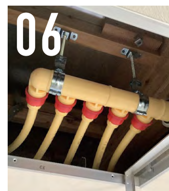
06 スプリンクラー配管
