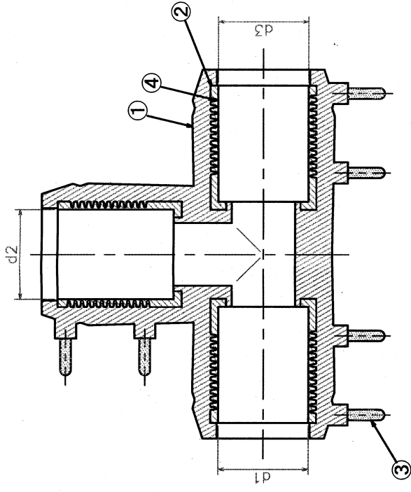
A-A 断面
