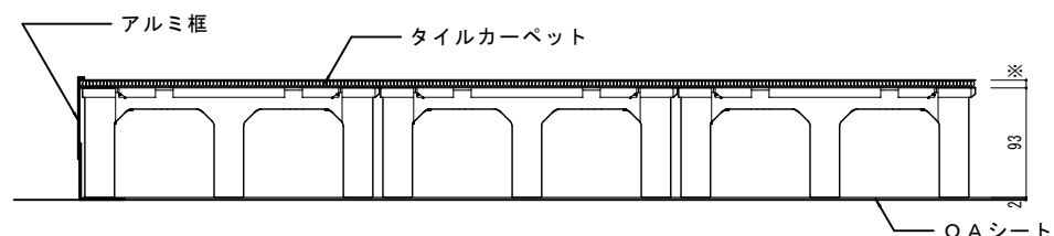
框部分断面詳細図 1/5
