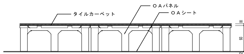
一般中央部断面詳細図 1/5
