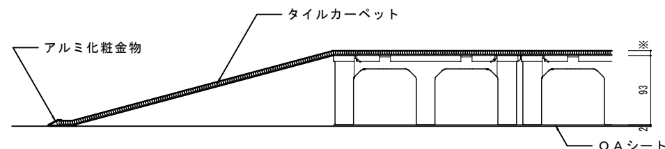
スロープ部分断面詳細図 1/5
