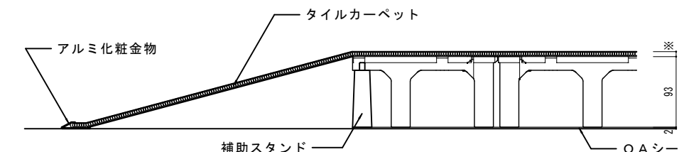
スロープ部分断面詳細図 1/5
