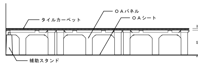
ボーダー部分断面詳細図 1/5
