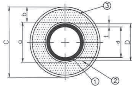
X-X'断面
