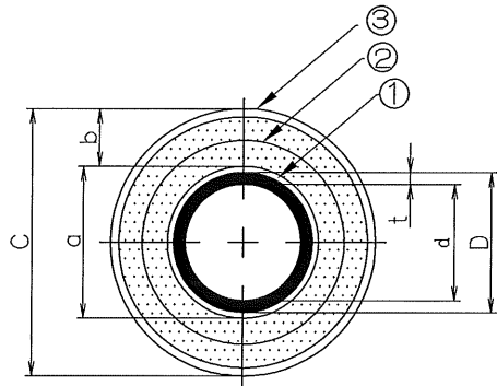
X-X'断面
