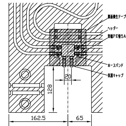
ヘッダー部詳細図 (1/5)
