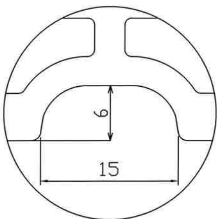
△B部拡大1:5
