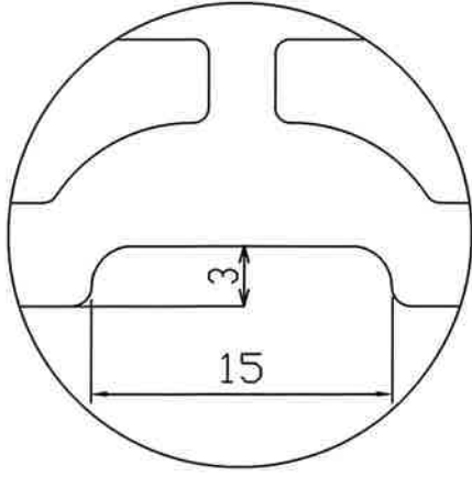
A部拡大1:5
