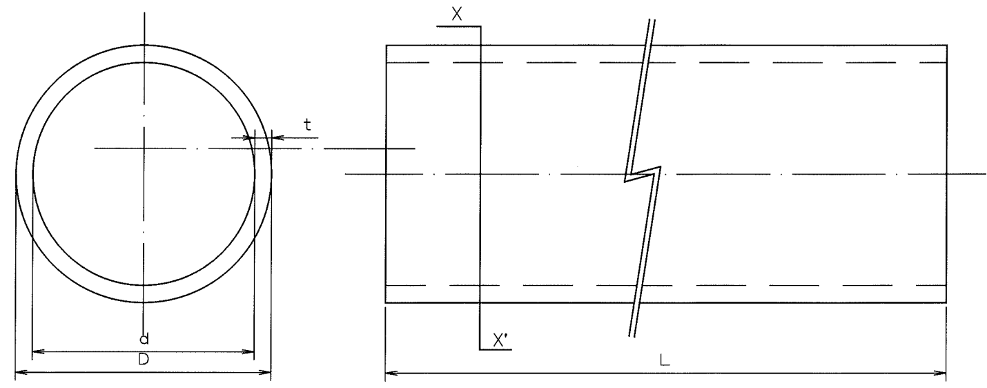
X-X' 断面図
