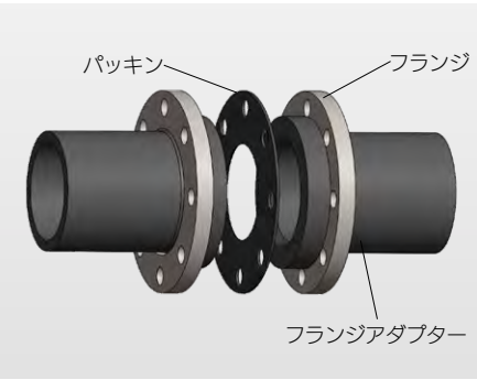
(組付け図)
