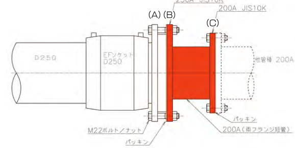
両フランジ短管が必要な場合の接続例
