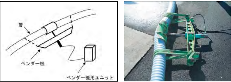
曲げ癖矯正
