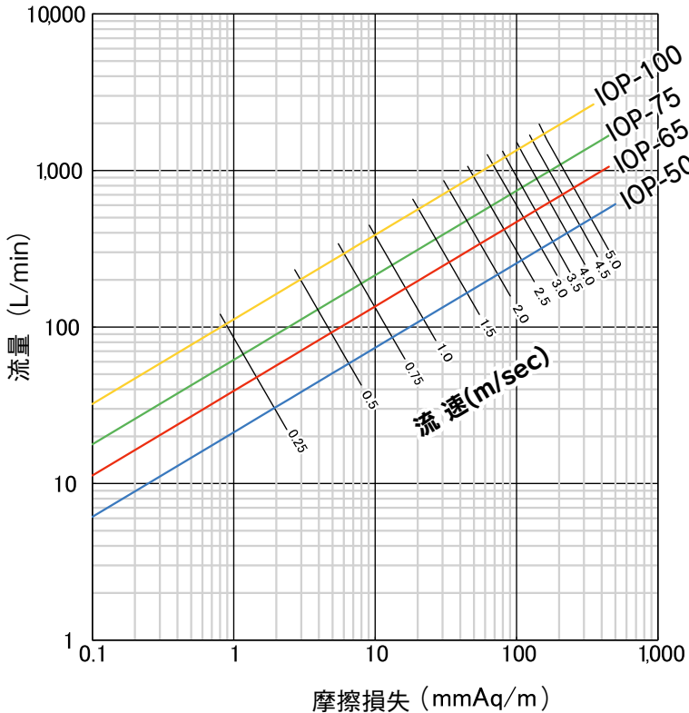
IOP-50 ～ IOP-100 流量線図
