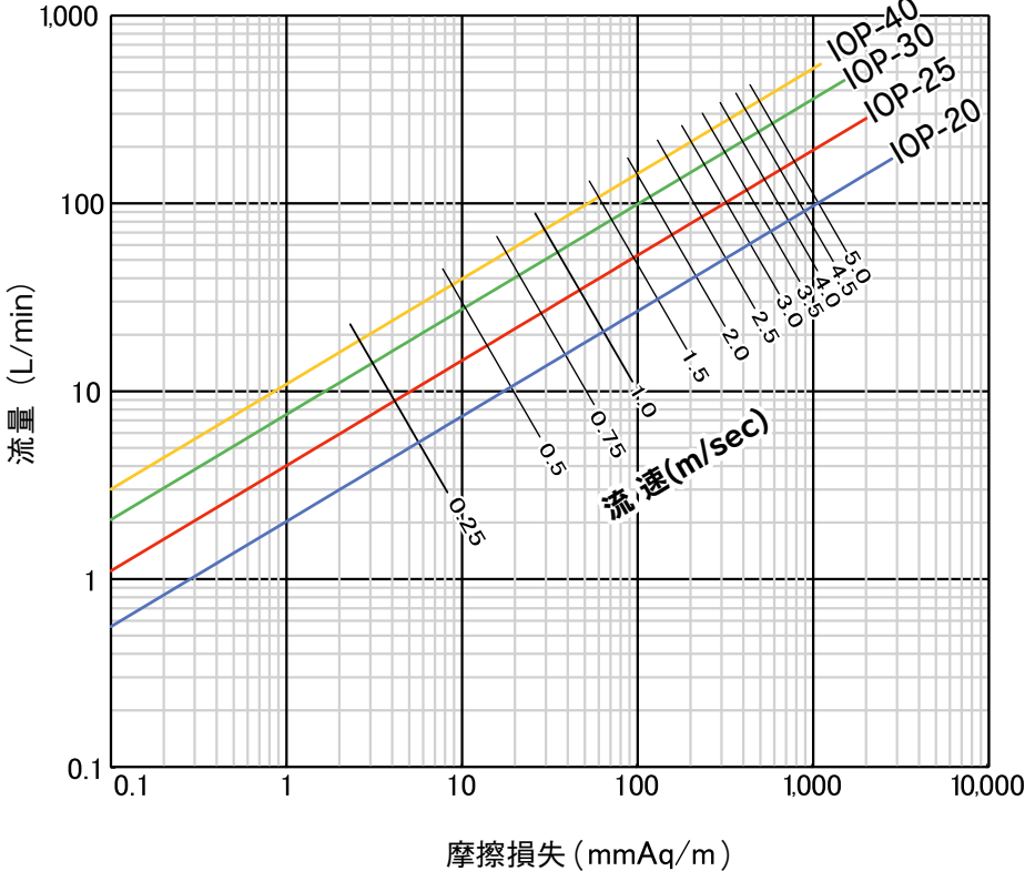
IOP-20 ～ IOP-40 流量線図
