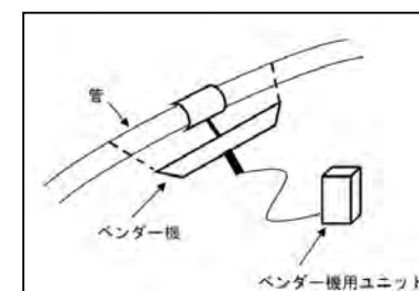
曲げ癖矯正
