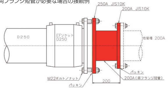
両フランジ短管が必要な場合の接続例
