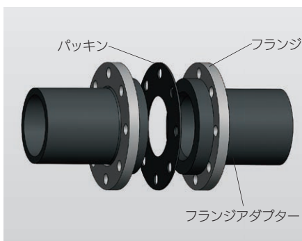
(組付け図)
